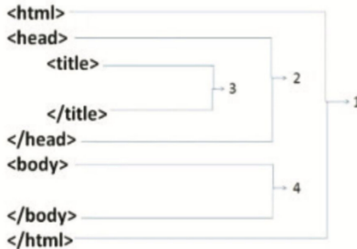
Gambar 1.1 Struktur Dasar HTML
